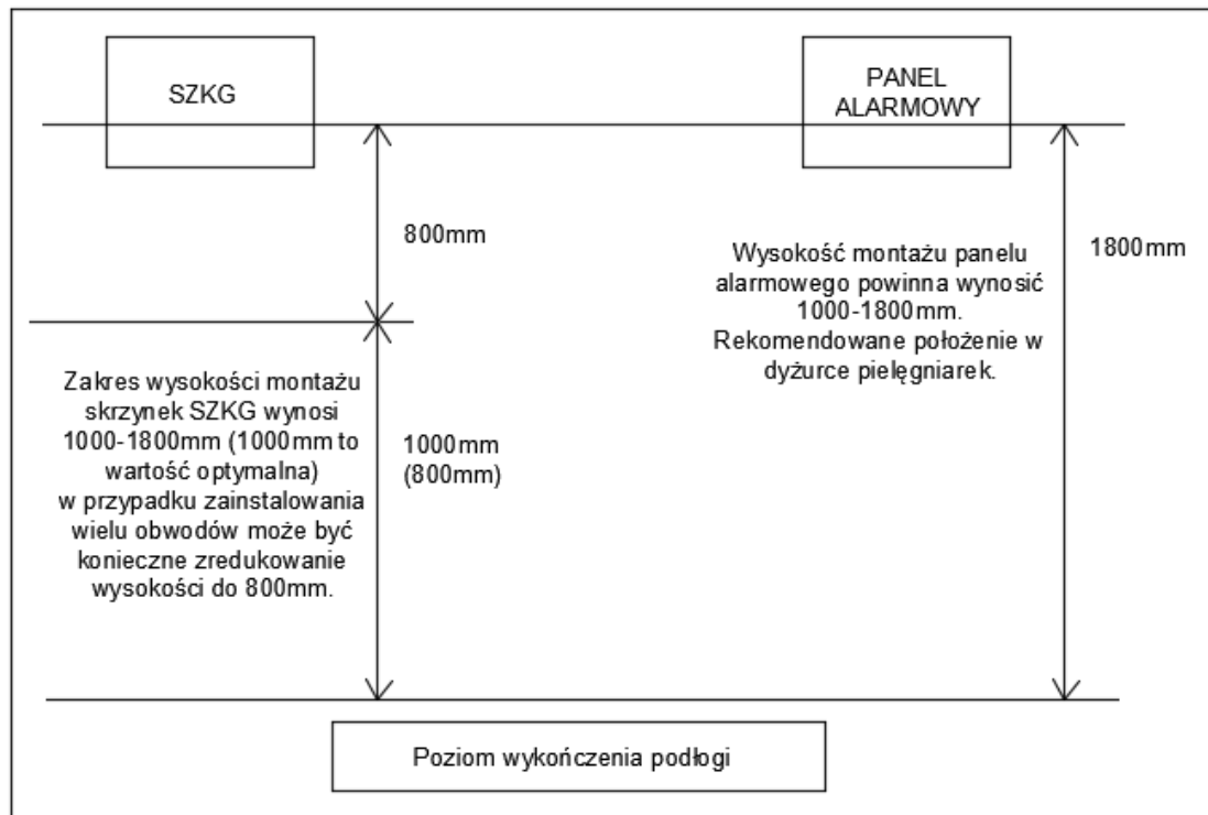
Rysunek 3 Wysokość montażu SZKG-SSGM
